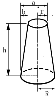
(カ) 截頭錐体
