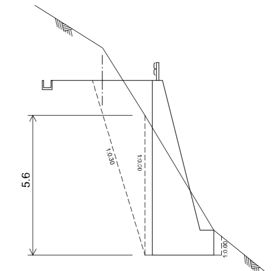
(6) 5.0m以上 (岩)
