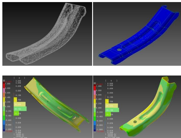
三次元形状測定（生産）
