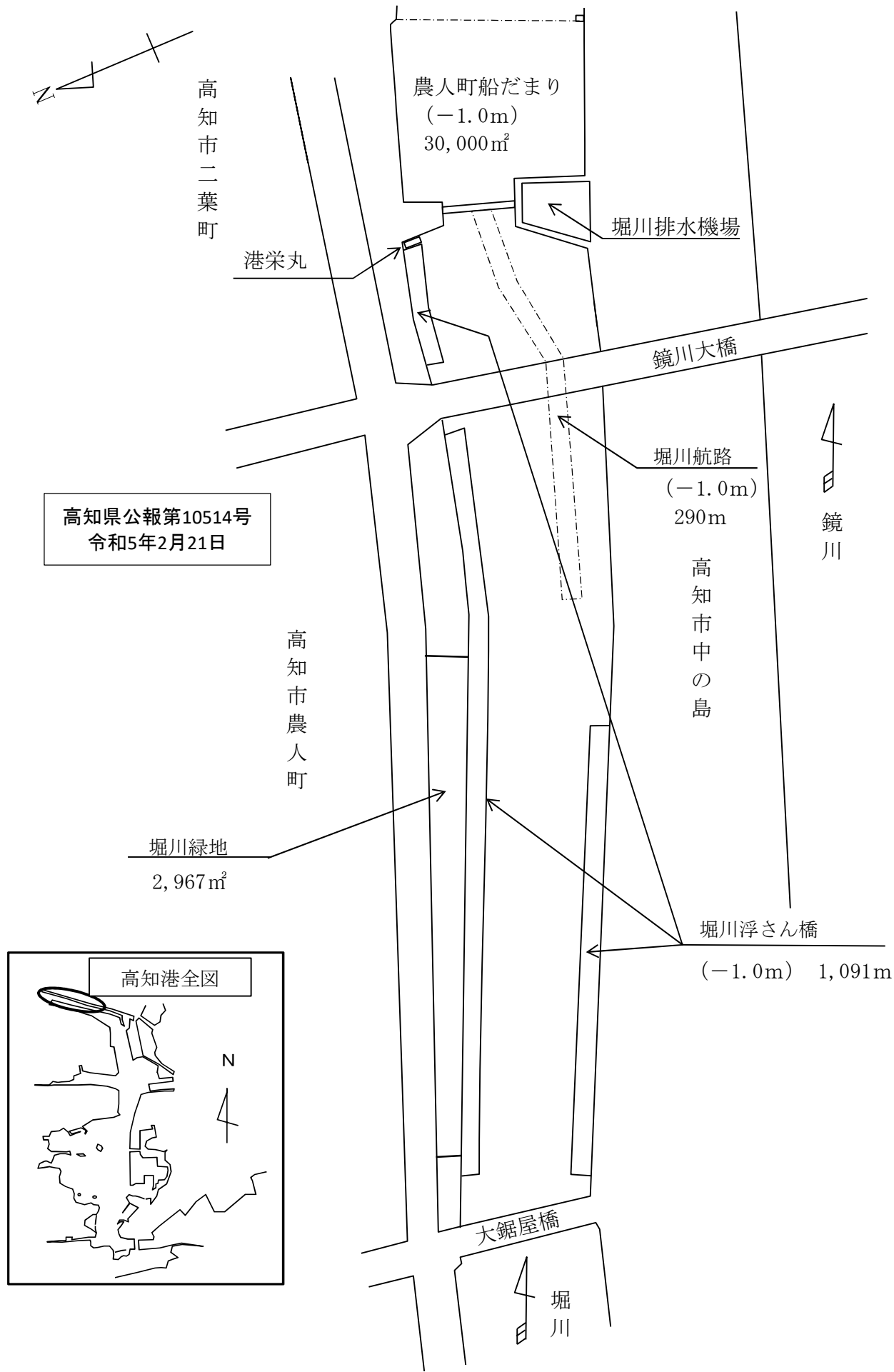
別図13 高知港堀川浮さん橋等の区域図
