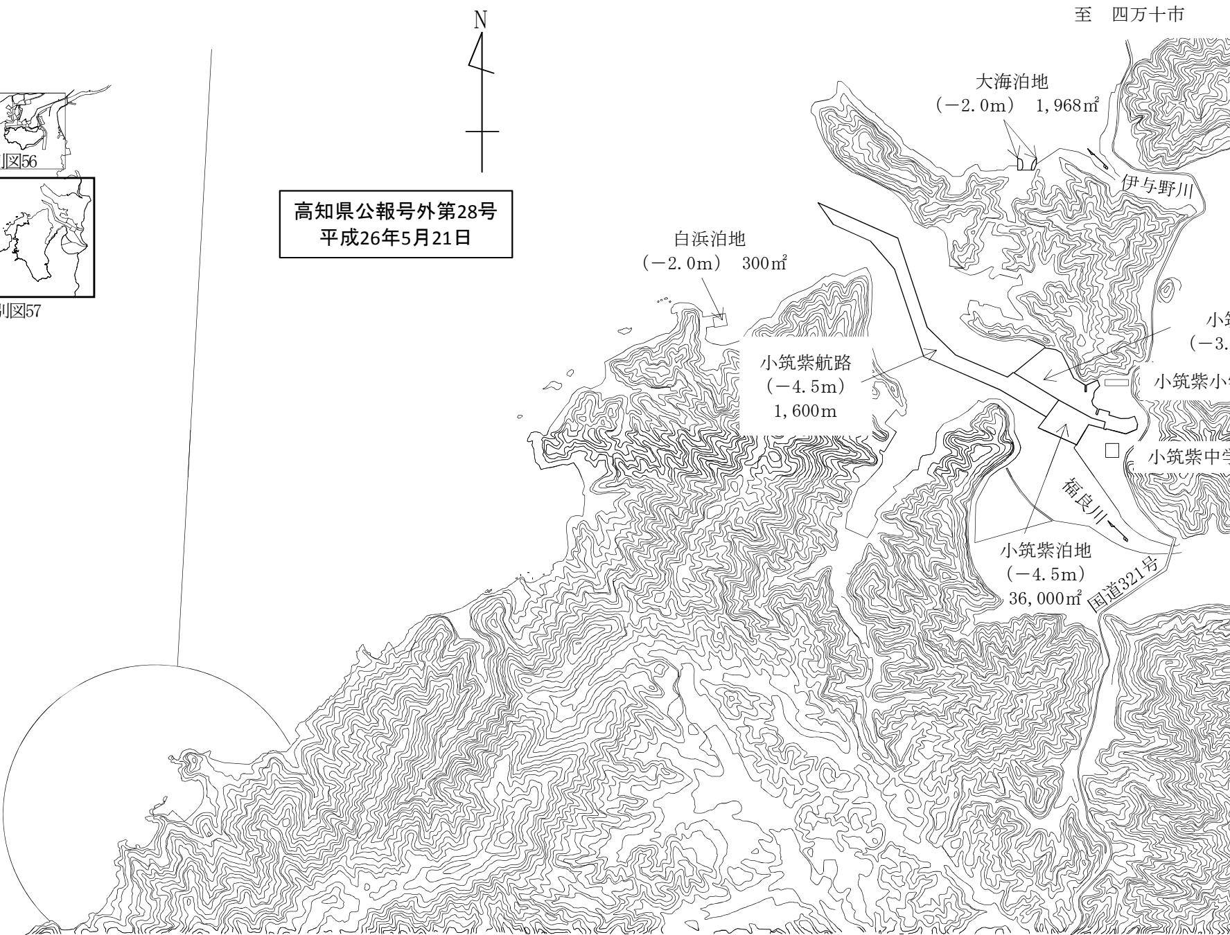
別図57 宿毛湾港小筑紫航路等の区域図
