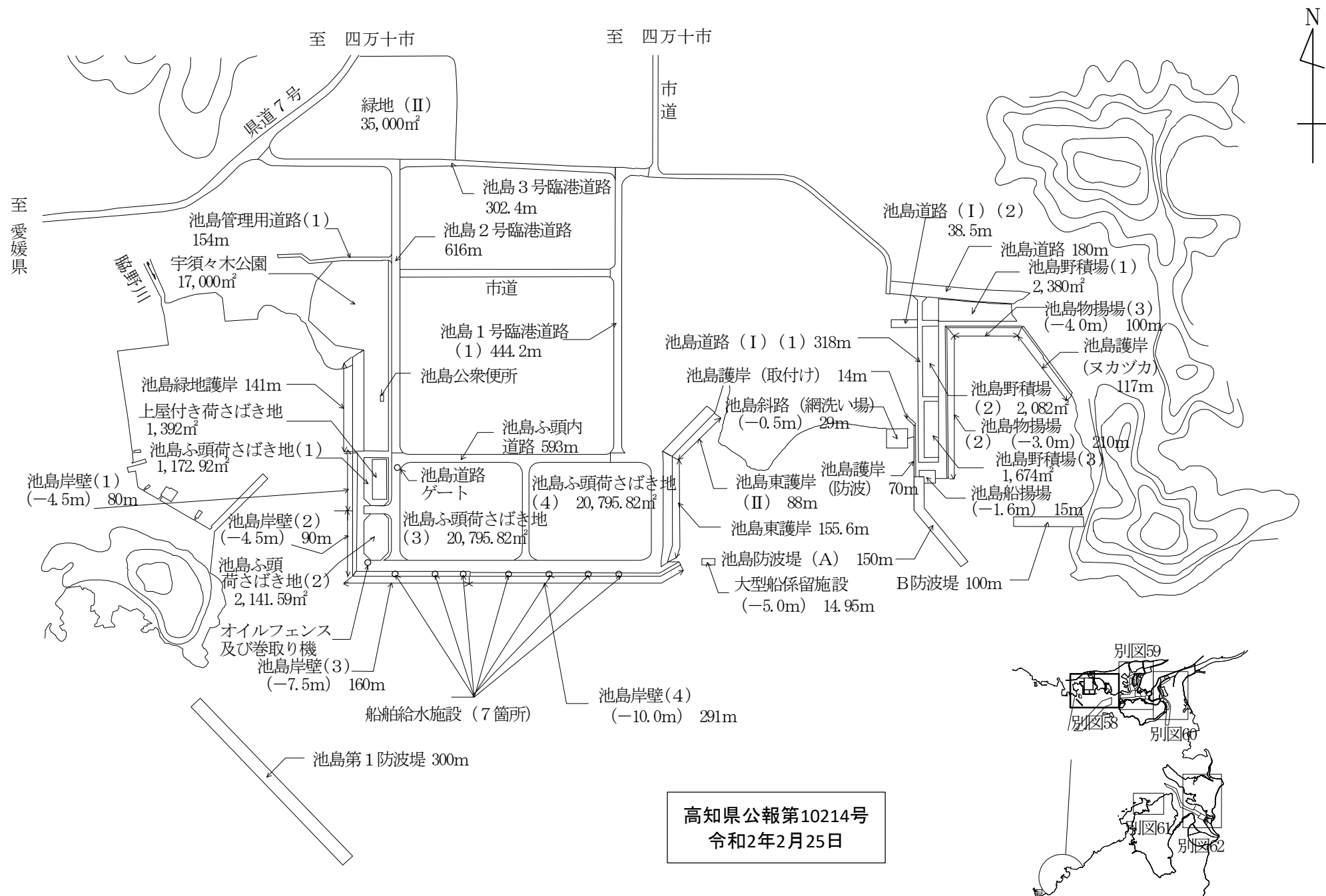
別図58 宿毛湾港池島岸壁等の区域図
