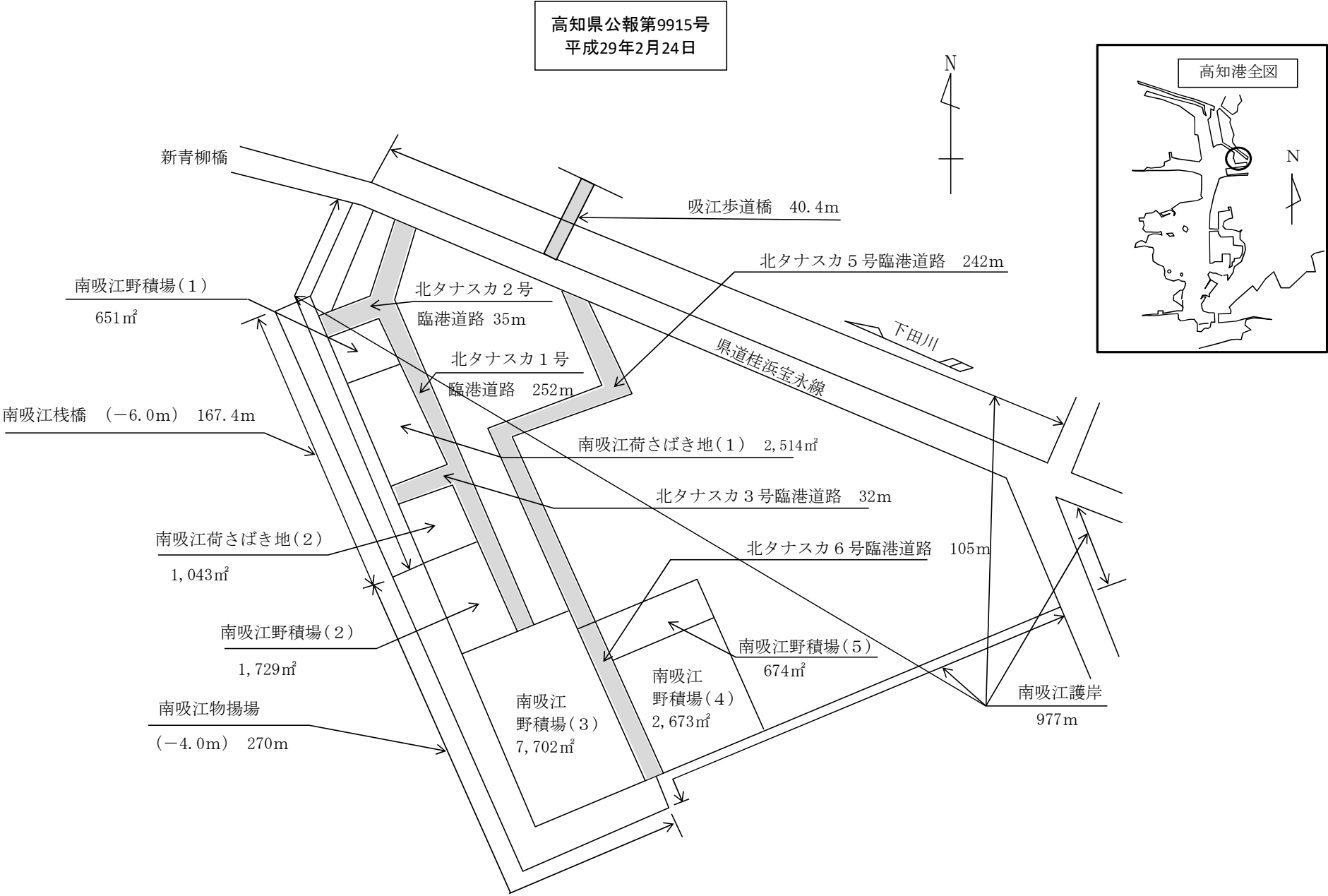
別図6 高知港南吸江物揚場等の区域図
