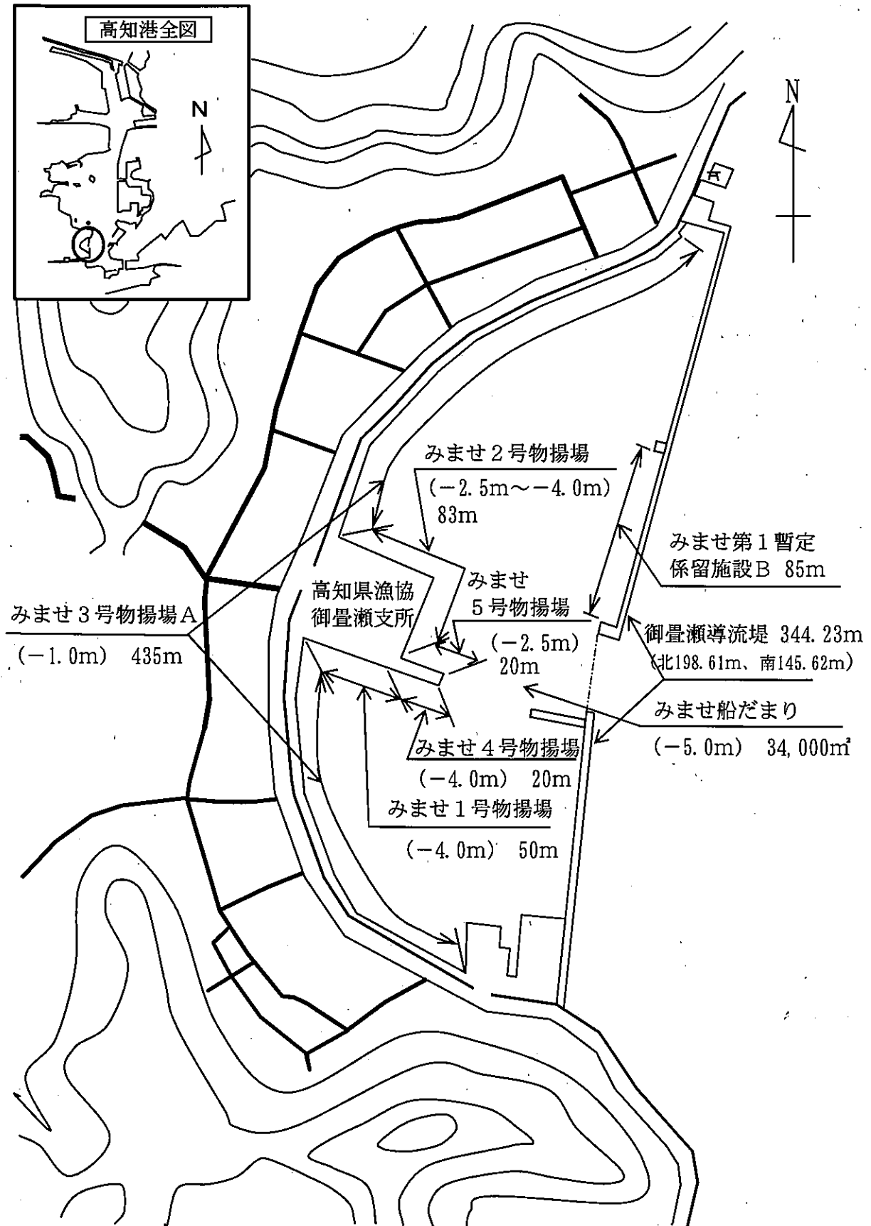
別図11 高知港御豊瀬物揚場等の区域図
