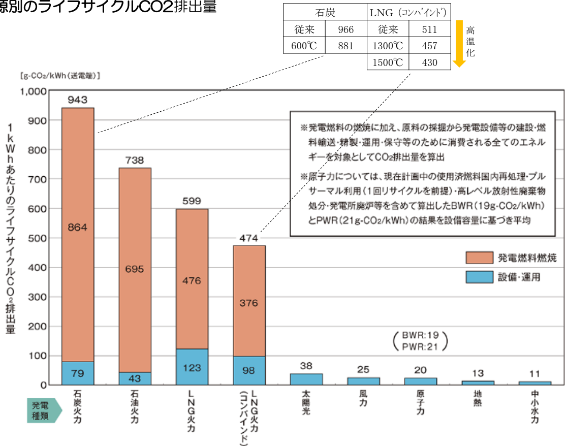
図⑫-7-1 各電源別のライフサイクルCO 2 排出量
