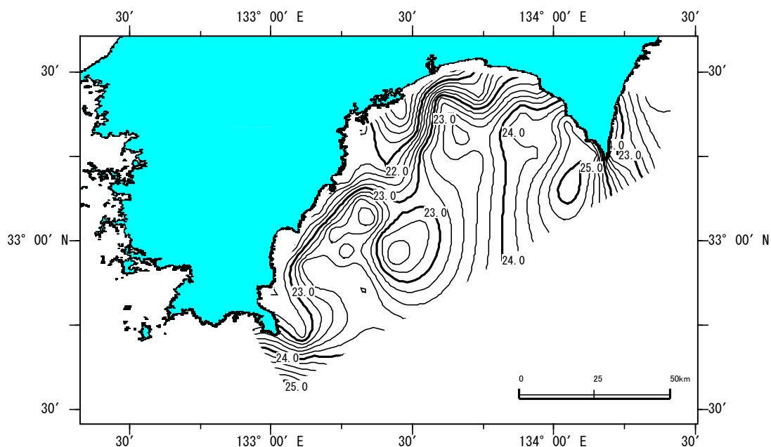
○深度0mの水温分布
