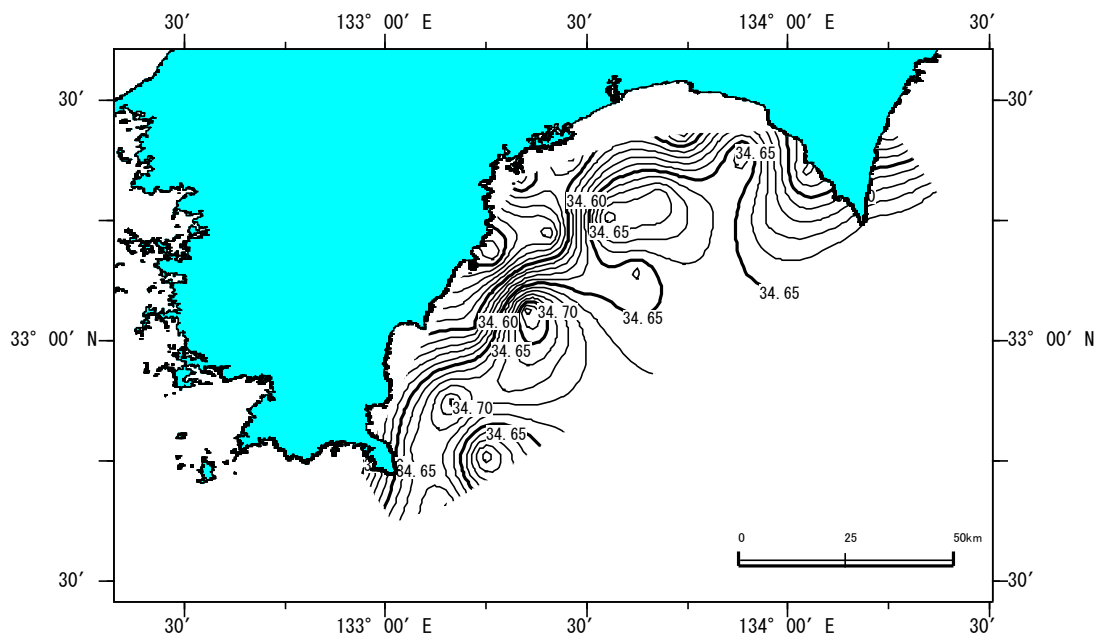
○深度 50m の塩分分布
