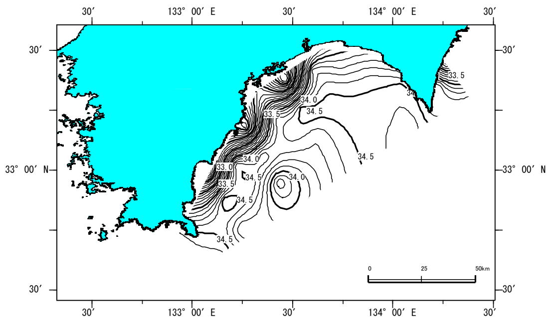
○深度0mの塩分分布
