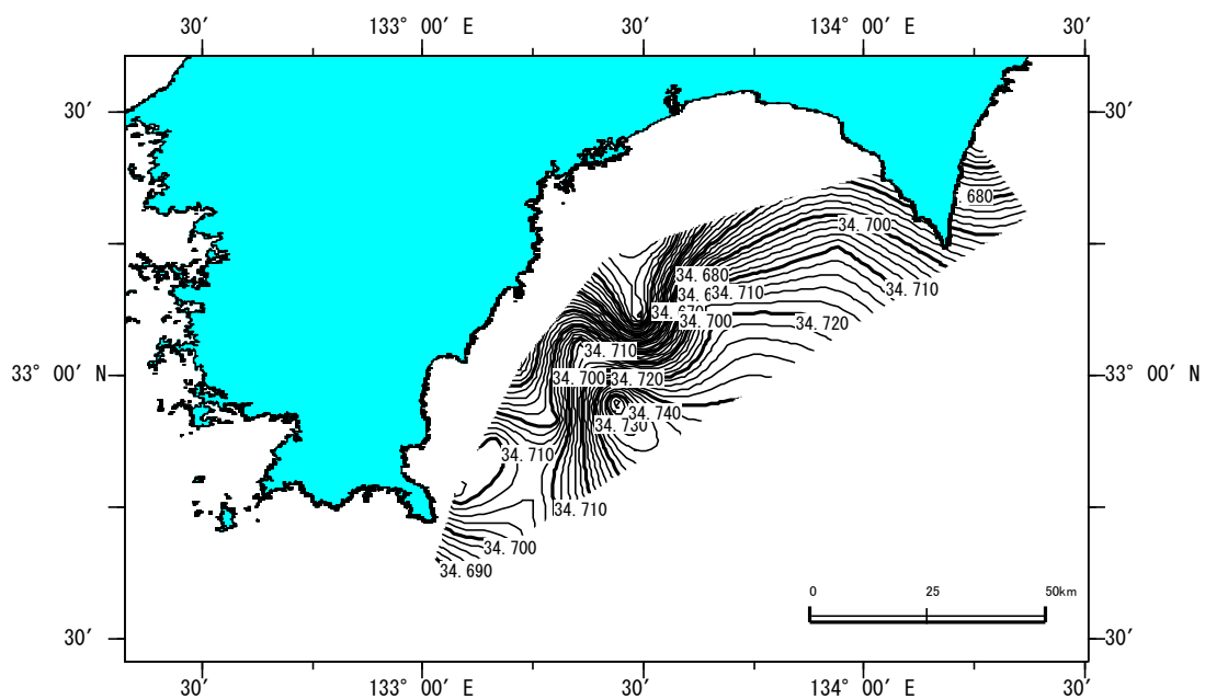
○深度 100m の塩分分布
