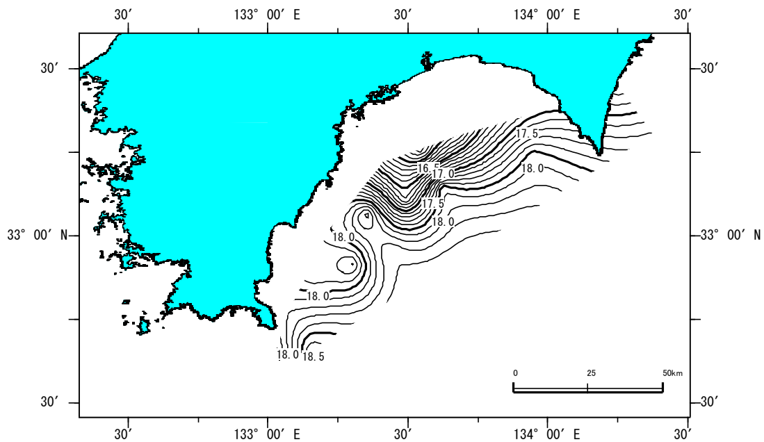
○深度 100m の水温分布
