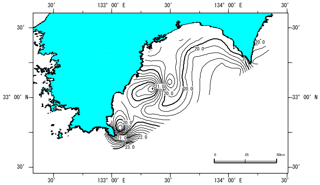
○深度 50m の水温分布
