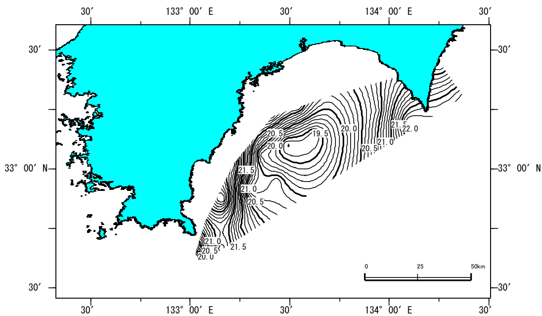
○深度 100m の水温分布 (単位: °C)
