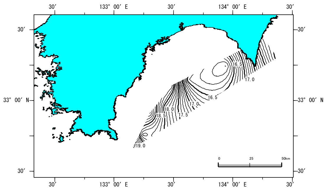
○深度 150m の水温分布 (単位: °C)
