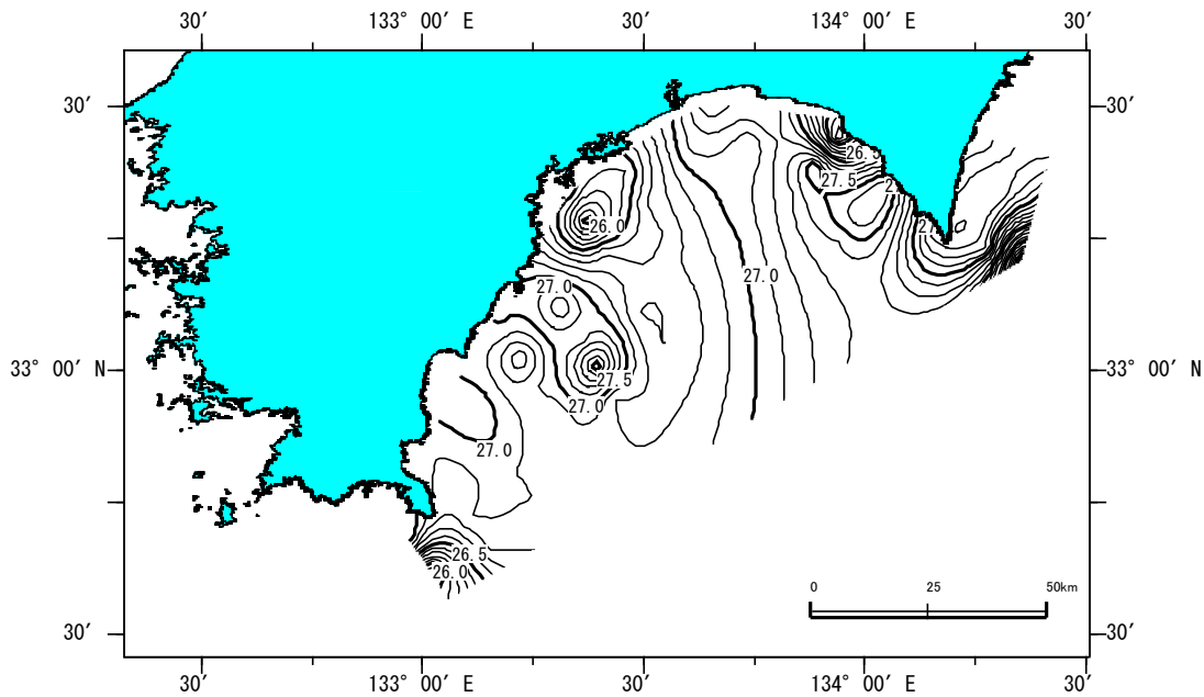
○深度0mの水温分布(単位:℃)
