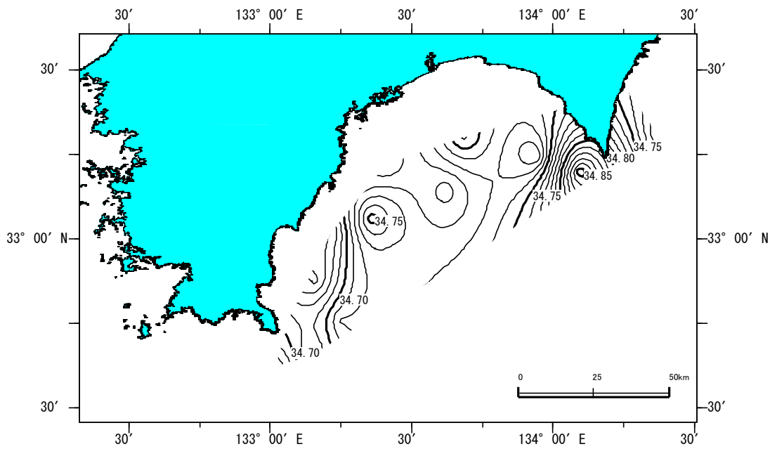
○深度 100m の塩分分布 (単位: ‰)
