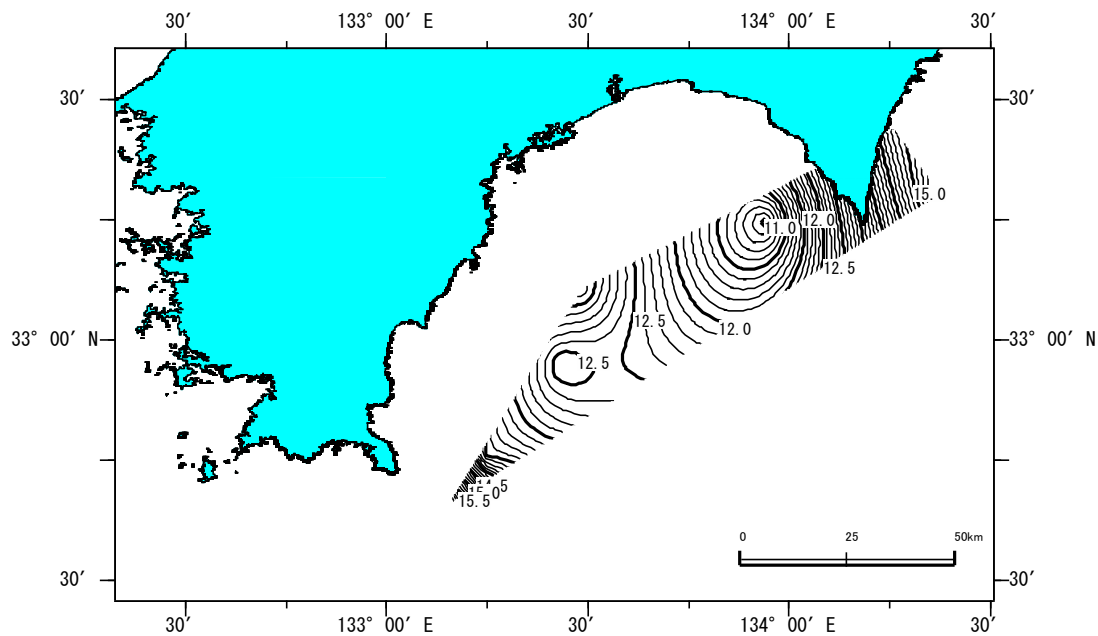
○深度 200m の水温分布 (単位: °C)
