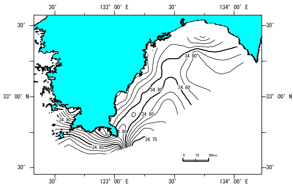
○深度 50m の塩分分布
