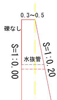
（ウ）帯工
