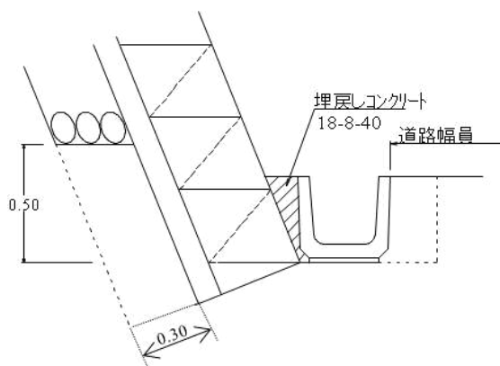
岩盤基礎
