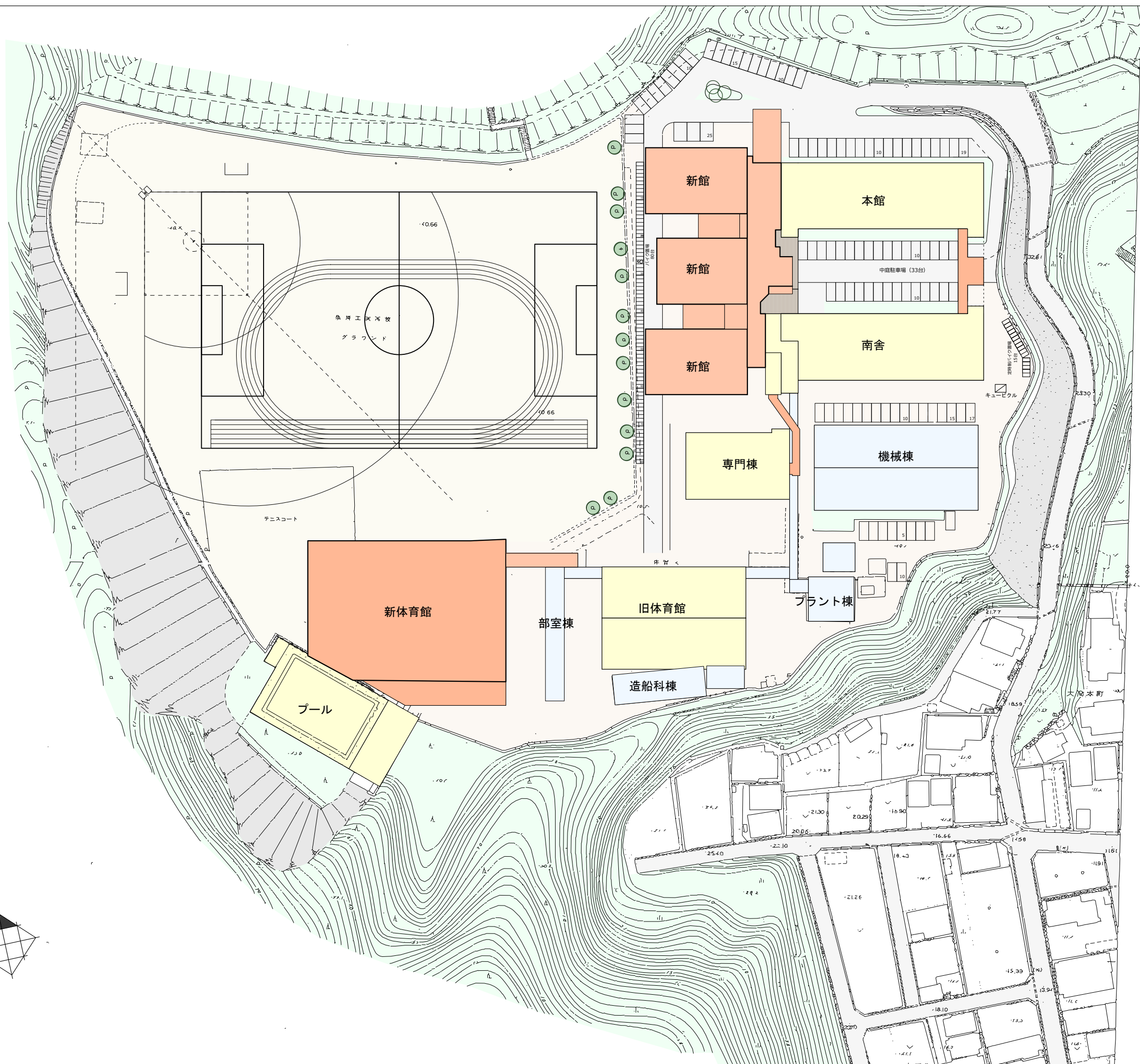
配置図 S=1/1000 (A3) 高吾地域拠点校基本設計委託業務
