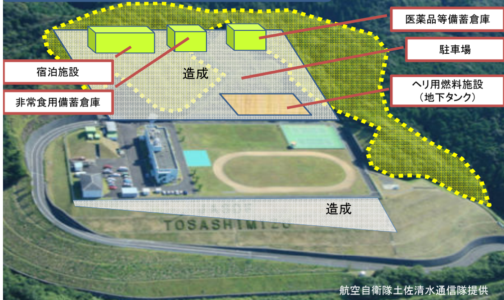
航空自衛隊土佐清水分屯基地ヘリポート関連施設配置イメージ図
