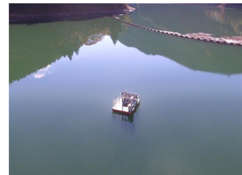
▲自動濁度計 全景
