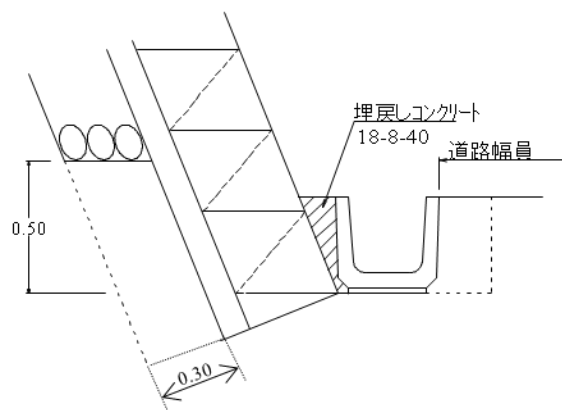
岩盤基礎
