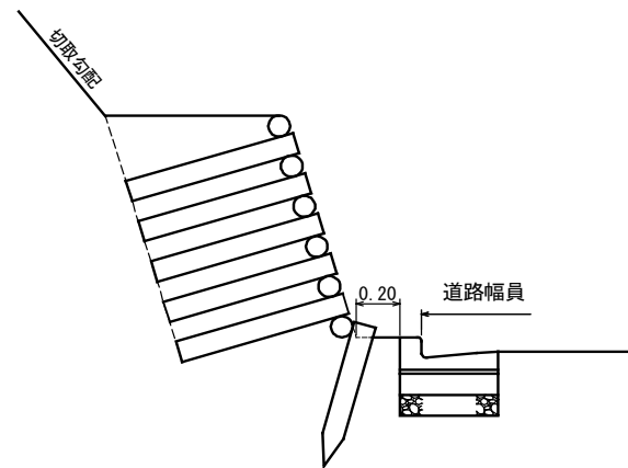
【丸太土留工】
