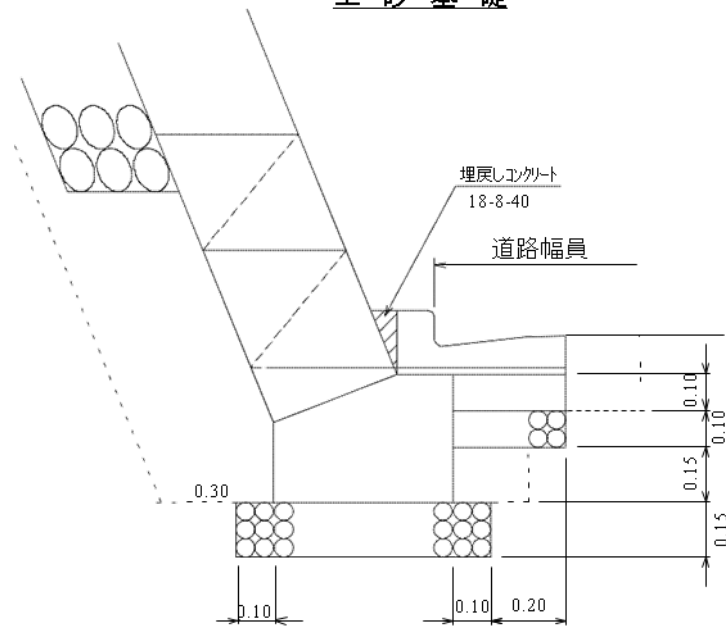
土砂基礎
