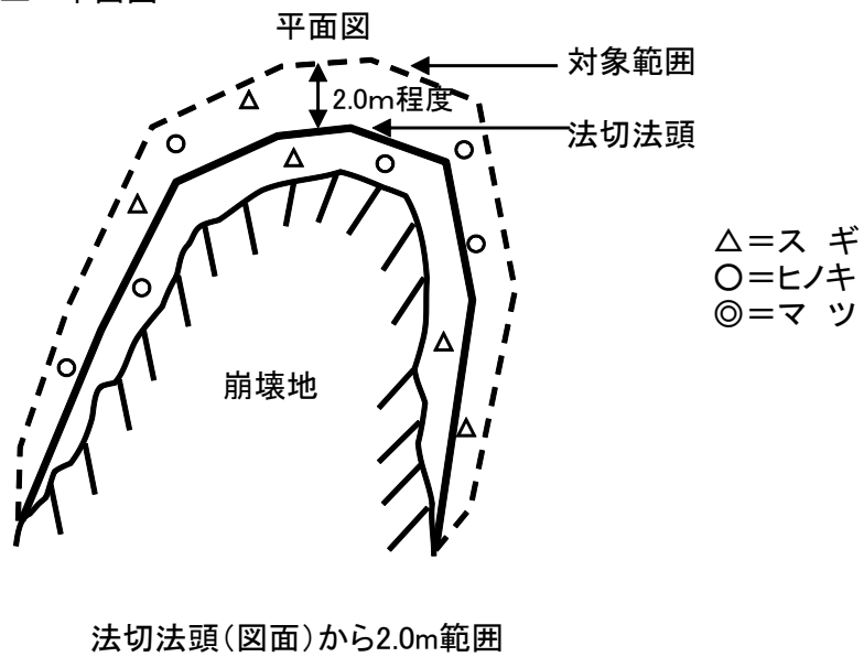
(2) 山腹工 平面図
