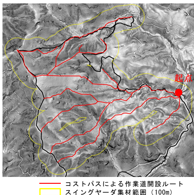
図3 スイングヤード集材の計画
