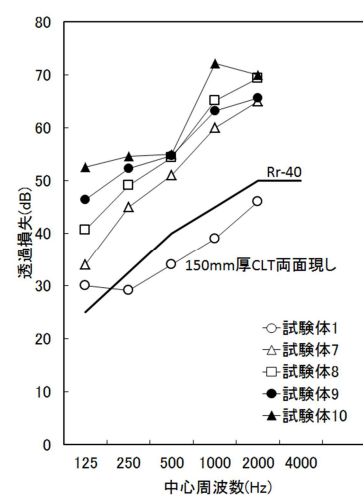
図 4 150mmCLT 厚両面仕様の結果
