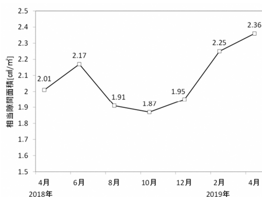
図 5 気密性能の季節変動
