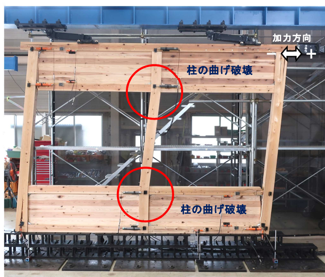
図 4 連結ラーメン構造試験体の変形状況
