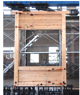
図1 ラーメン構造による耐力壁
