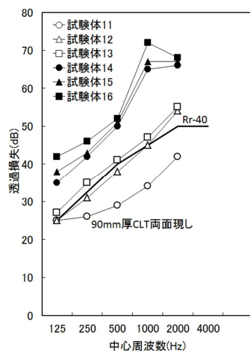
図 5 90mm 厚 CLT 片面仕様の結果
