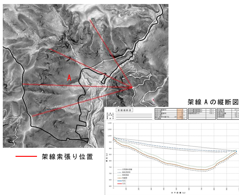
図4 架線集材の計画
