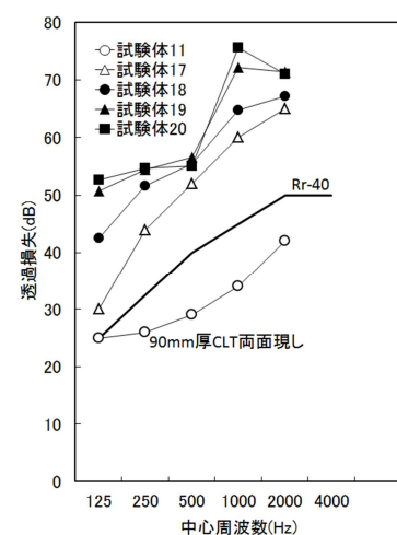
図 6 90mm 厚 CLT 両面仕様の結果
