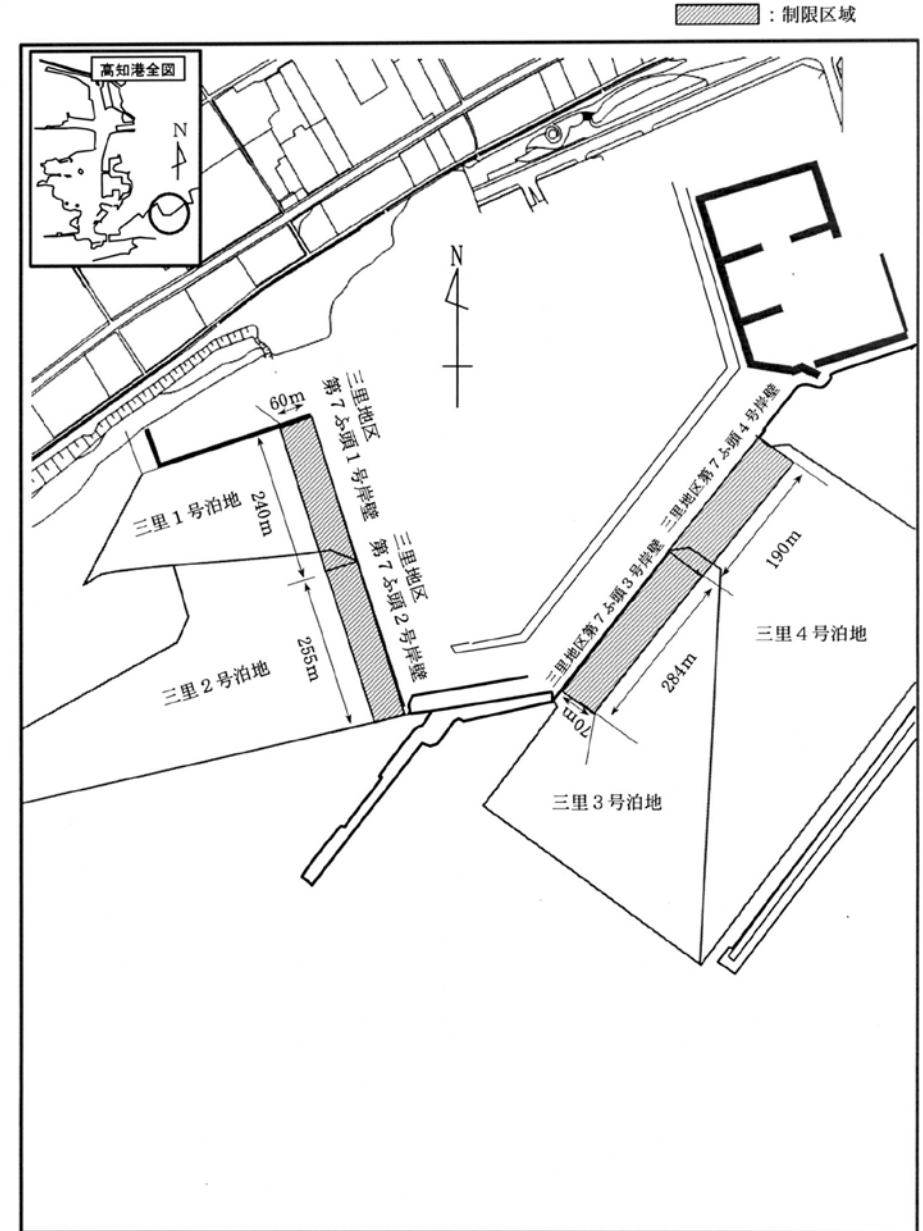
別図3 高知港三里1号泊地、三里2号泊地、三里3号泊地及び三里4号泊地内の制限区域図
