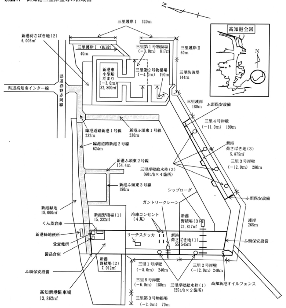
別図17 高知港三里岸壁等の区域図
