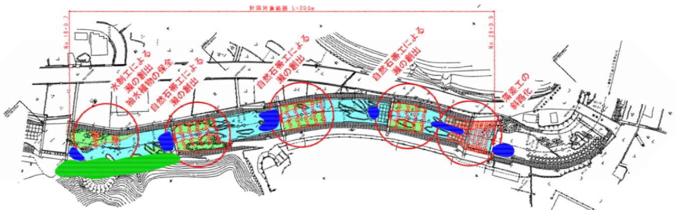
計画平面図
