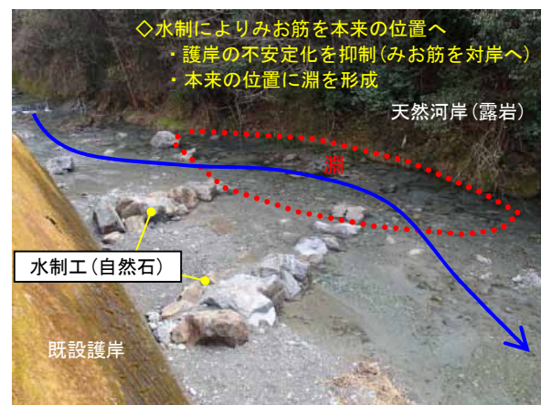
水制設置か所（工事完了直後）
