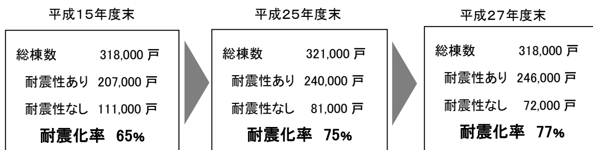
図表2-4 住宅の耐震化の状況
