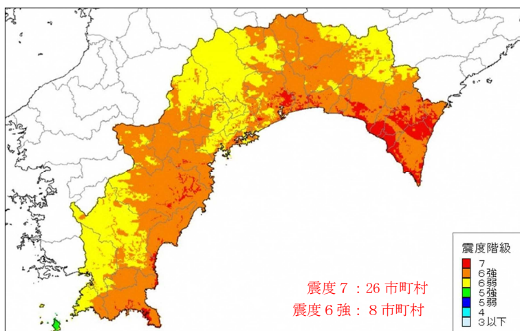
図表1-2 震度分布図(L2)
