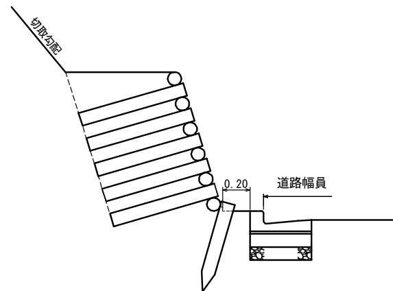
【丸太土留工】
