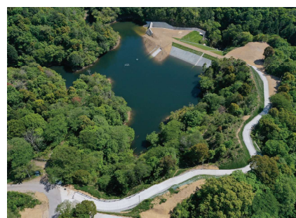
伊尾木地区農村災害対策整備 竜王池改修工事 四国開発 株式会社
