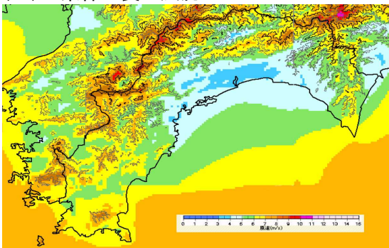
出典：NEDO 局所風況マップ
