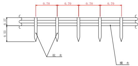
正面図
