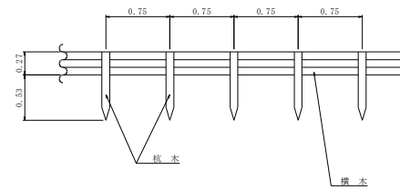
正面図
