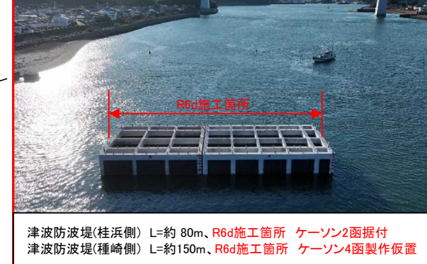
津波防波堤(桂浜側) 堤頭部・堤幹部(R7.1撮影)
