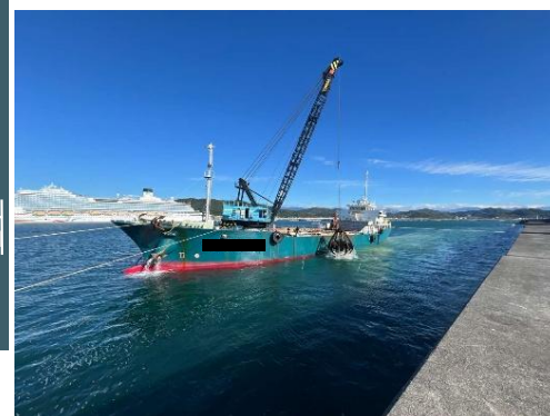
①防波堤(東第一)(直轄施工) 腹付工(R7.10撮影)
