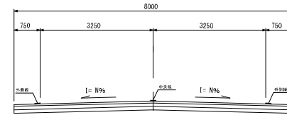
【幅員構成】
