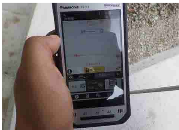
杭ナビによる出来形検測
