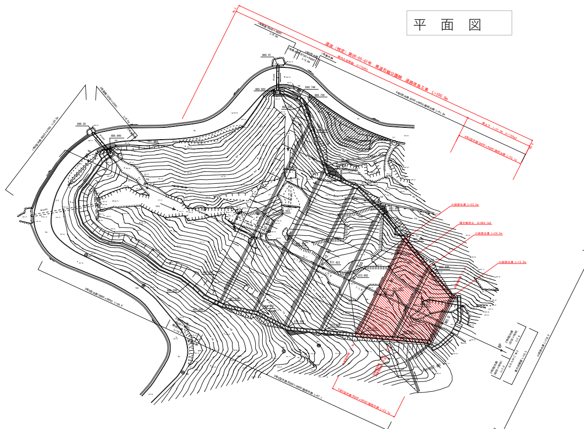
平 面 図
