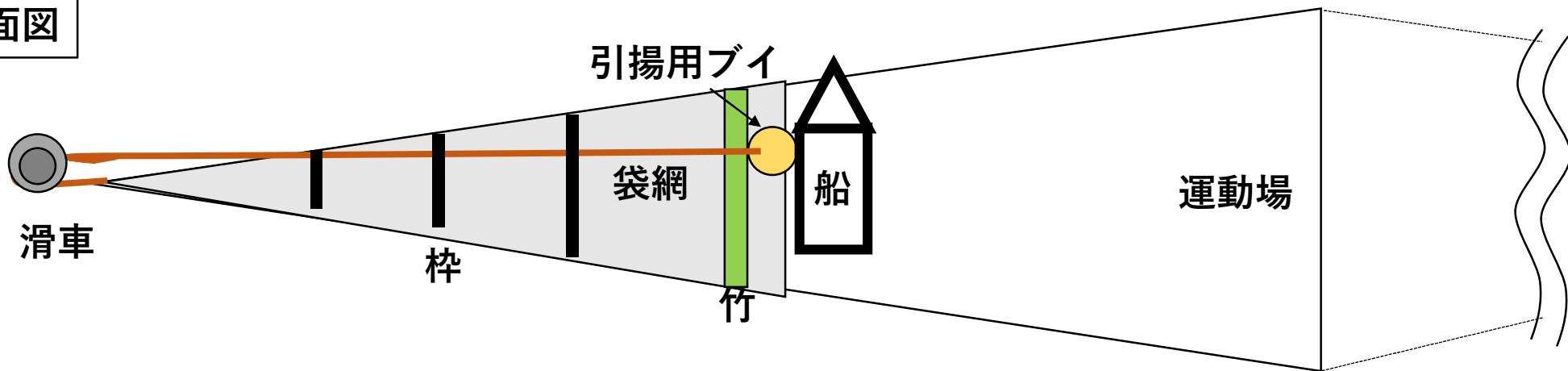
側面図
