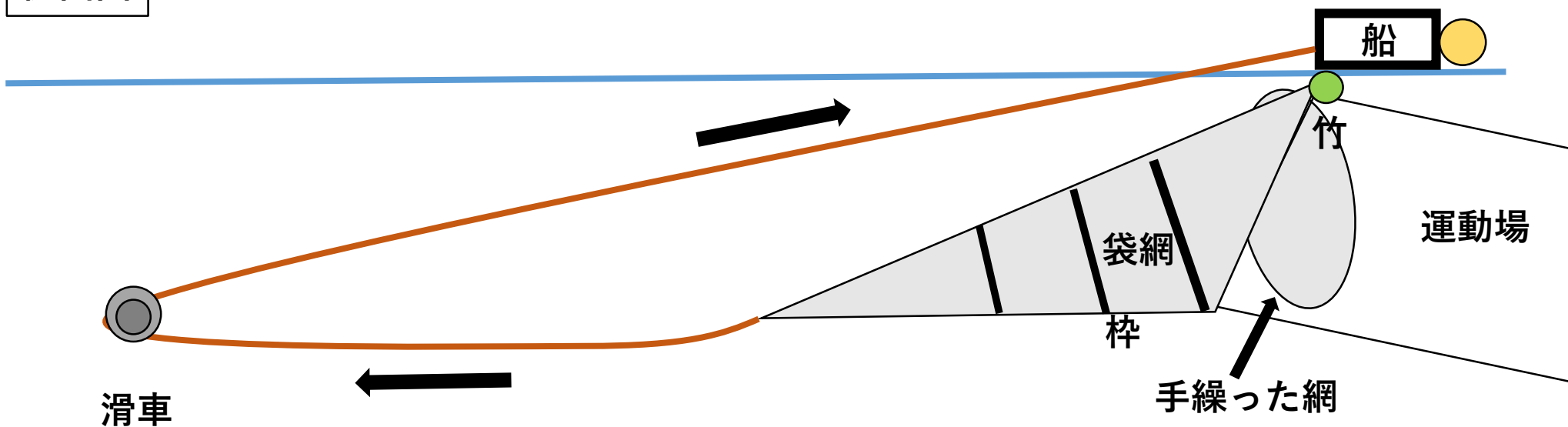
側面図
