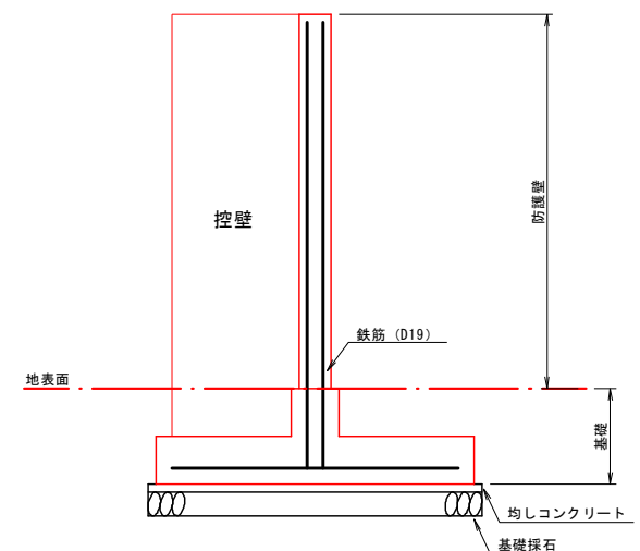
標準断面（控壁部）
