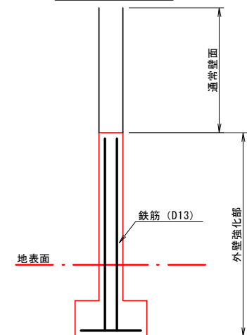
標準断面
