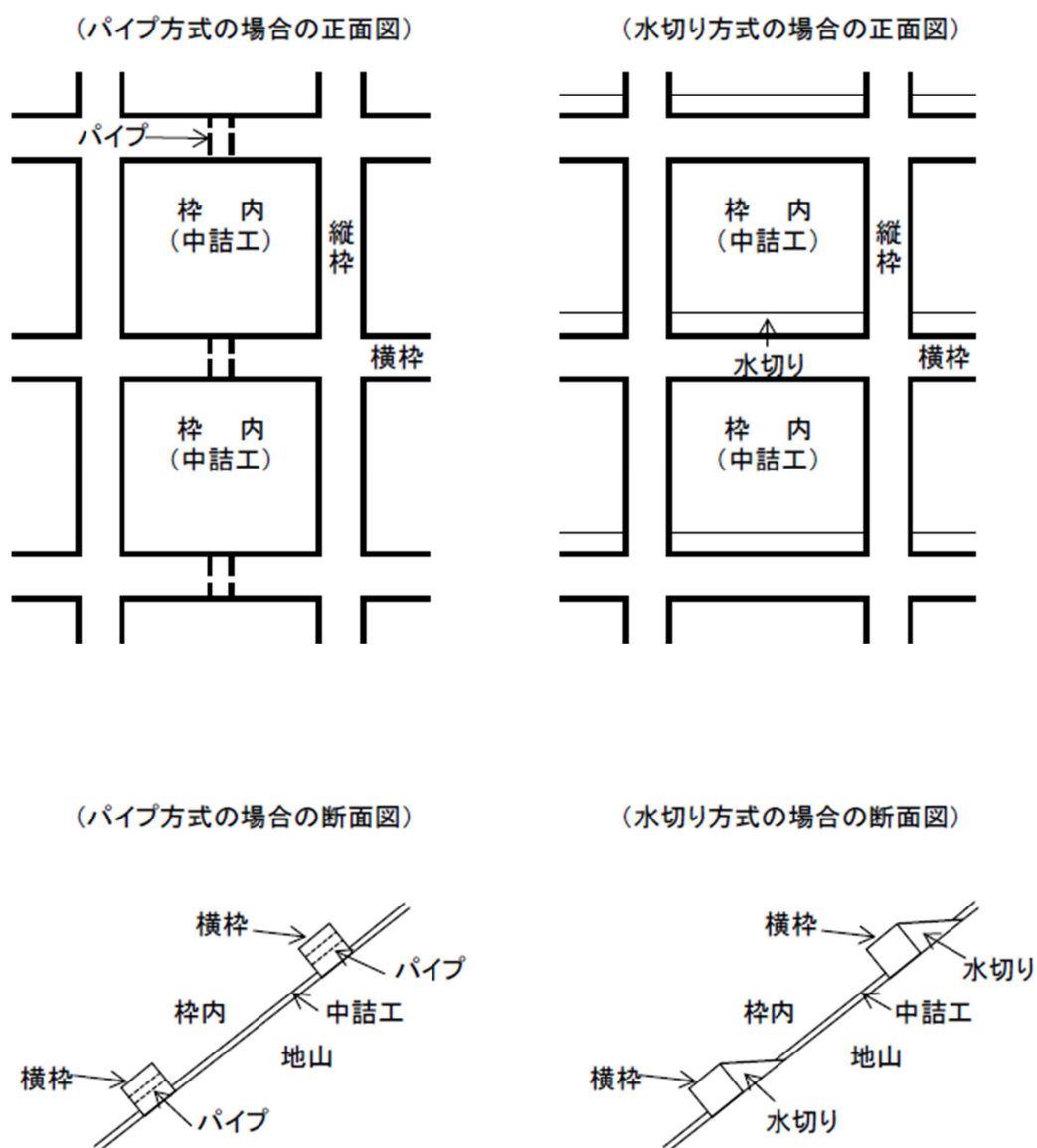
現場吹付法枠工の概念図
