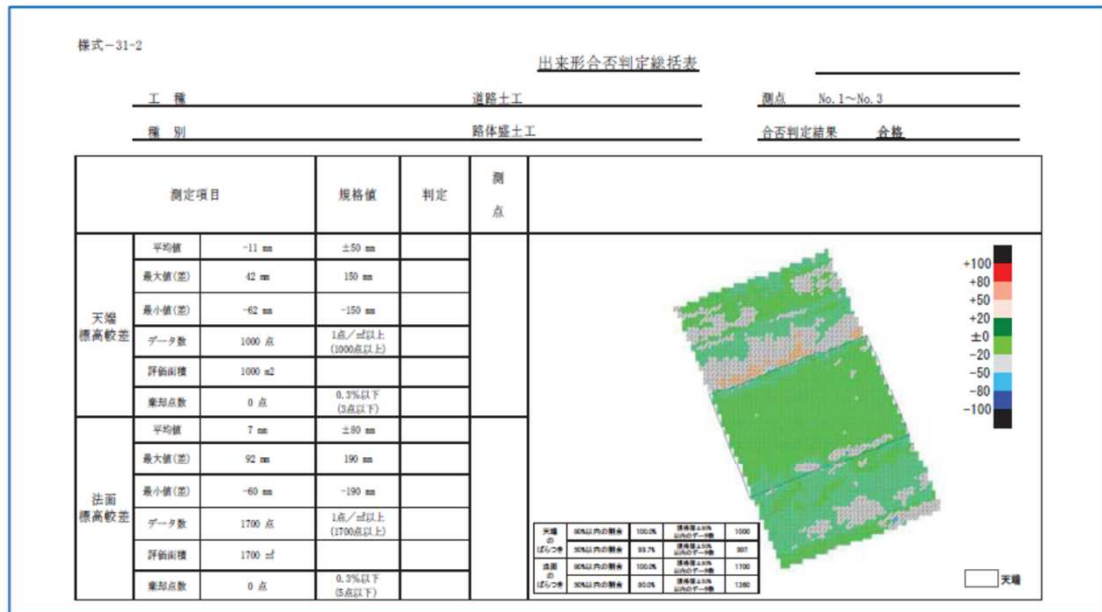
図 5-2 出来形管理図表 作成例 (合格の場合)
