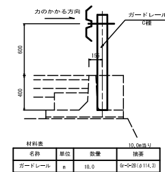
ガートルール S=1:20 (Gr-C-2B)
