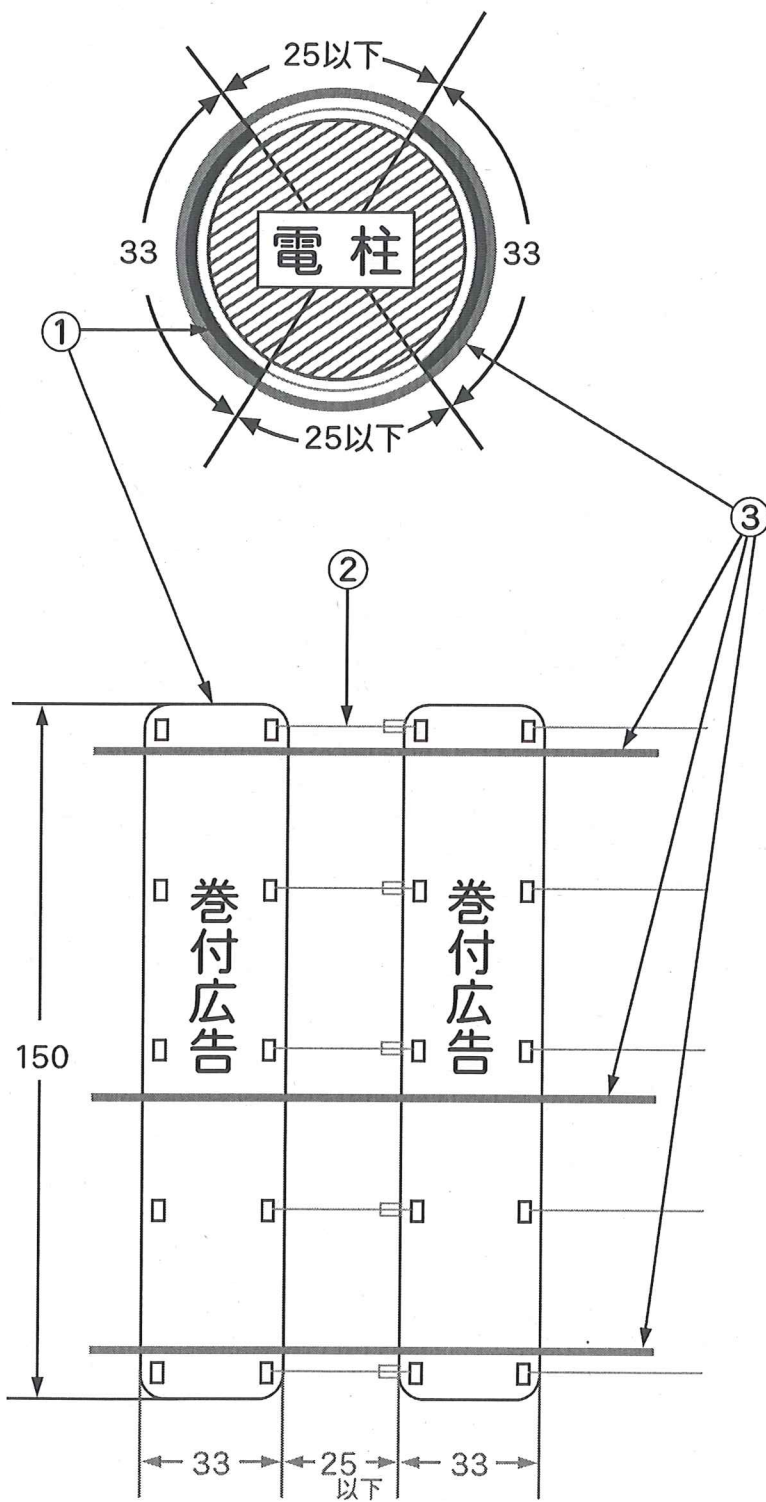
図5 巻付広告取付使用図2
