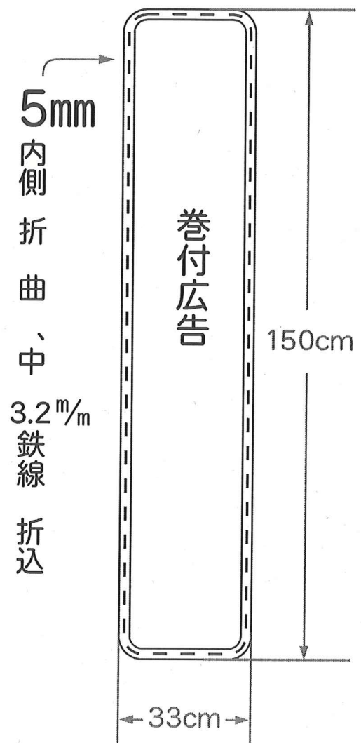
図1 巻付広告規格図
