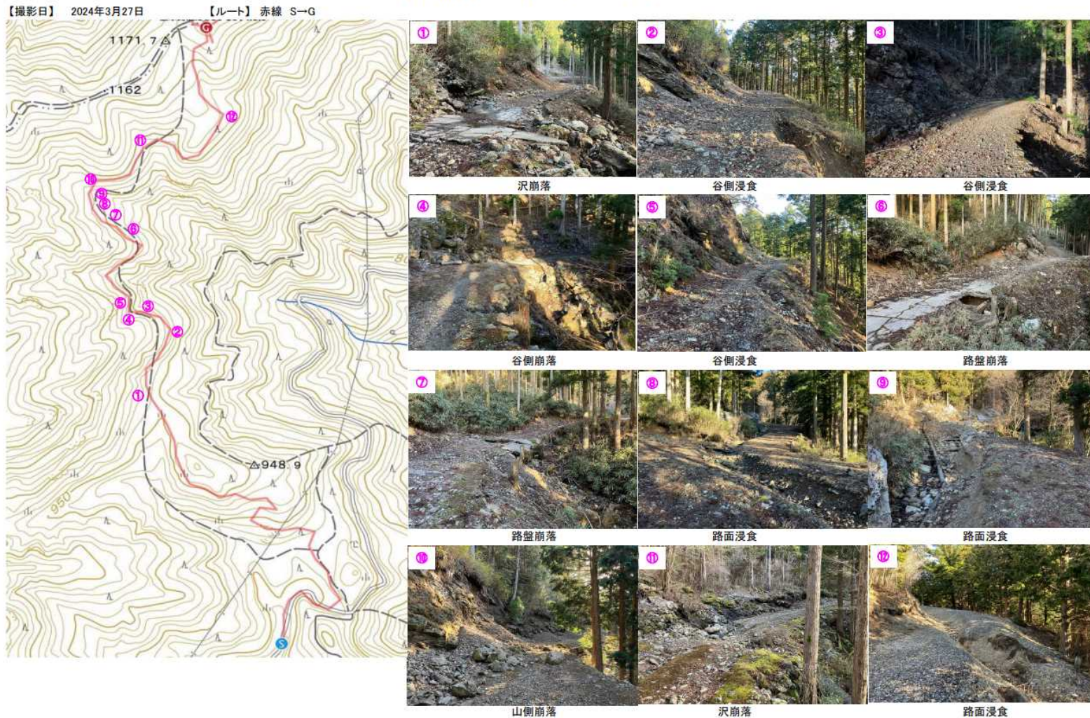
香美市香北町河野 作業道現況写真
