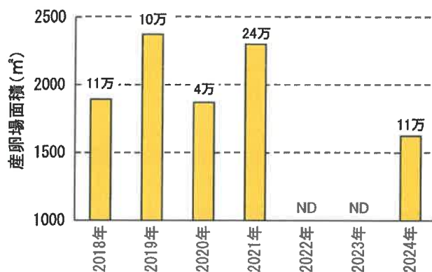
図 6-3 産卵所面積の経年変化 図中数値は秋季のアユ推定生息数
