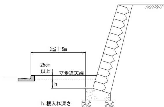
図 根入れの深さ_擁壁前面に L 字型側溝を設ける場合
