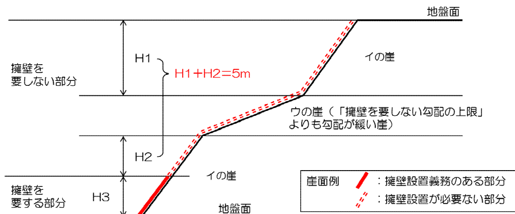
図 崖の途中で角度が変化する場合の擁壁の必要性の考え方
