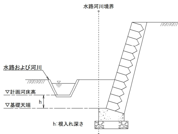
図 根入れの深さ_水路、河川に接している場合
