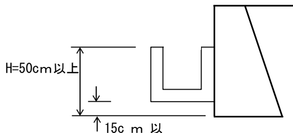
(d) 既存施設に隣接して設置する場合
