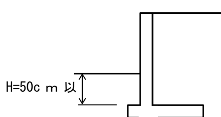
(c) 逆 T 型擁壁
