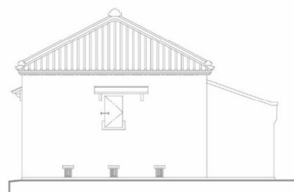
[ 南立面図 ]
