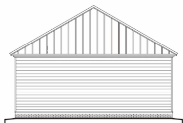
[北立面図]
