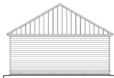
[南立面図]
