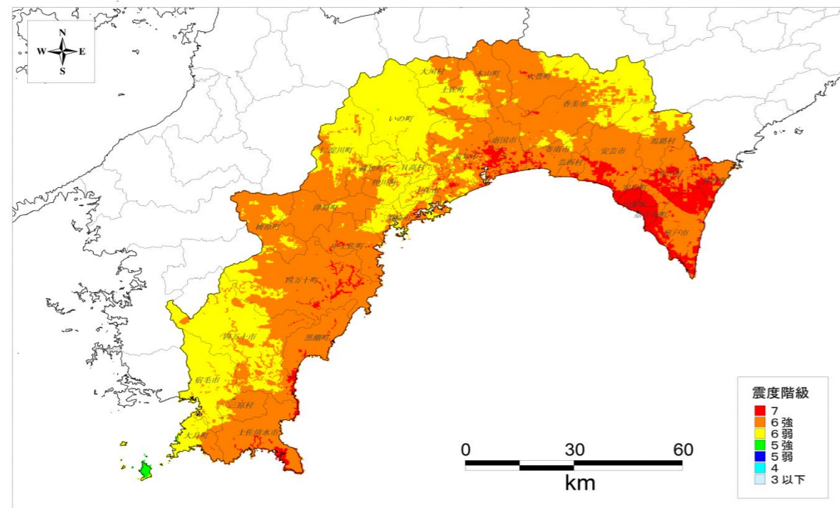
図表 2-1 震度分布予測図（複数ケースの重ね合わせ）
