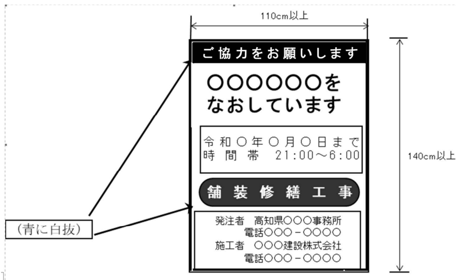
図1-2 標示板の例
