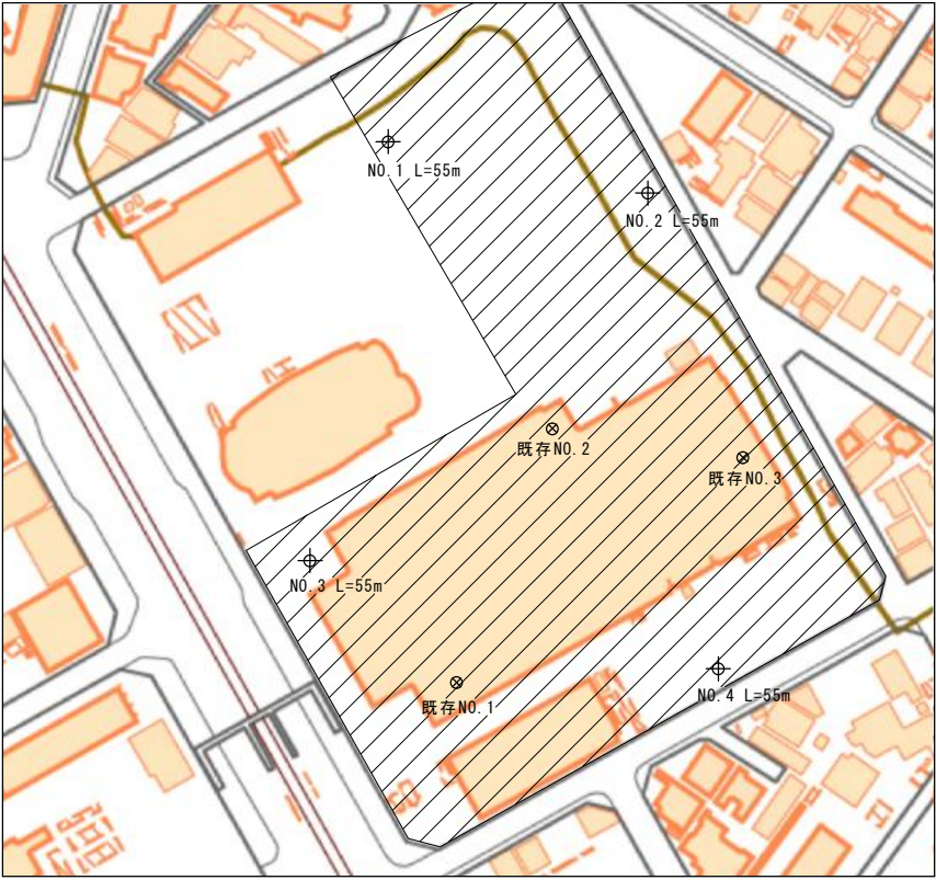
配置図
