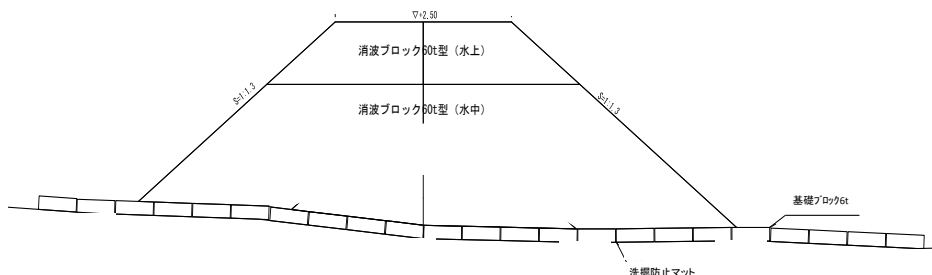
標準断面図
