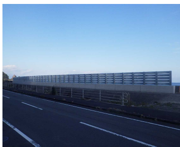
鹿岡海岸（越波防護柵）
