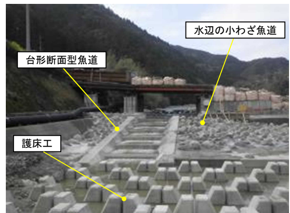
魚道工施工状況
