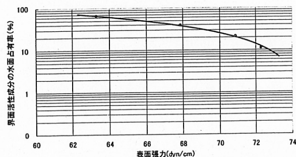
図4-11 水面における表面張力と界面活性成分分子占有率の推定(黒尊川トロ淵)
