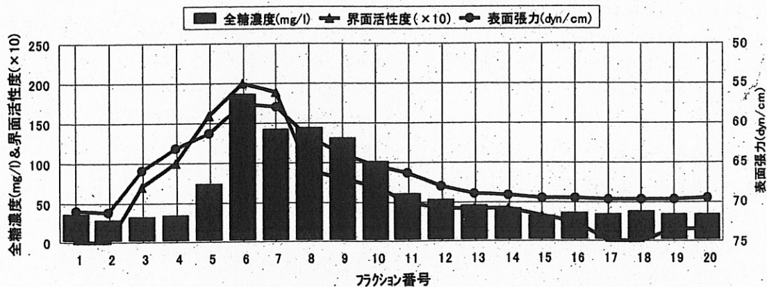
図5-10 弱陰イオン交換カラム (DEAE) フラクシヨンの性状パターン (サンプル：黒尊川上流トドロ淵の泡沫水)
