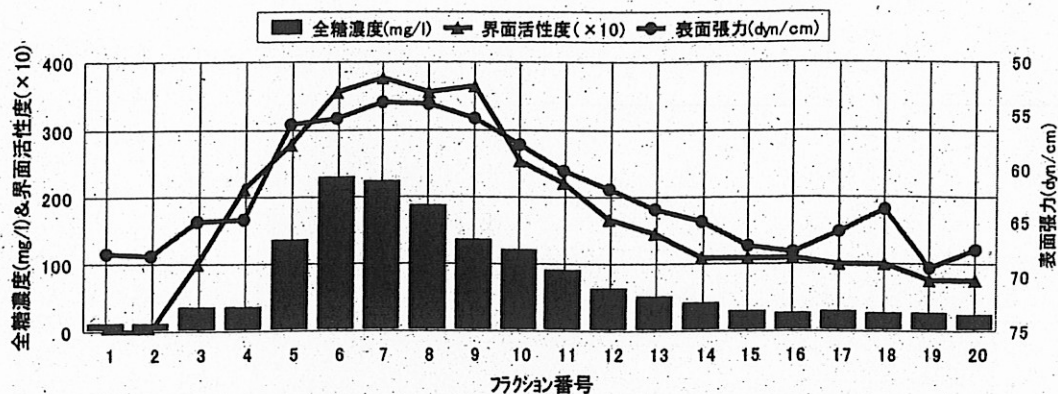
図5-8 弱陰イオン交換カラム (DEAE) フラクシヨンの性状パターン (サンプル：四万十川十和村広瀬泡沫水)
