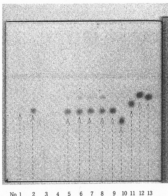
図5-7 薄層クロマト結果(3)
