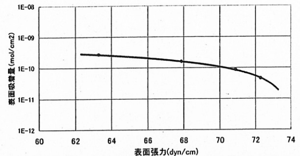
図 4-9 水面における表面張力と界面活性成分表面吸着量の関係（黒尊川トドロ淵）
