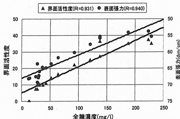
図5-12 DEAE 溶離フラクション性状の相関 (四万十川と和村広瀬) (全糖濃度—界面活性度・表面張力)
