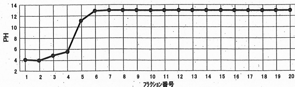
図5-11 弱陰イオン交換カラム (DEAE) フラクシヨンの性状パターン (PH) (サンプル：黒尊川上流トドロ淵の泡沫水)
