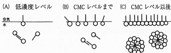
図 2-4 水中における界面活性物質の濃度と存在形態
