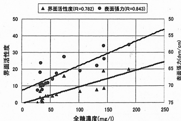
図5-13 DEAE 溶離フラクション性状の相関 (黒尊川トドロ淵) (全糖濃度—界面活性度・表面張力)
