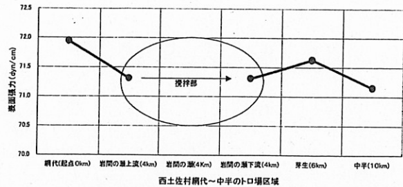
図4-4 トロ場における流水面の表面張力変化状況(H12. 4.13/強風)
