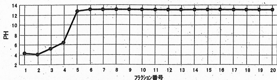
図5-9 弱陰イオン交換カラム (DEAE) フラクシヨンの性状パターン (PH) (サンプル：四万十川十和村広瀬の泡沫水)
