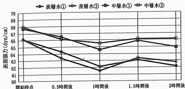
図4-1 静置状況下における河岸凹部の表面張力の経時変化
