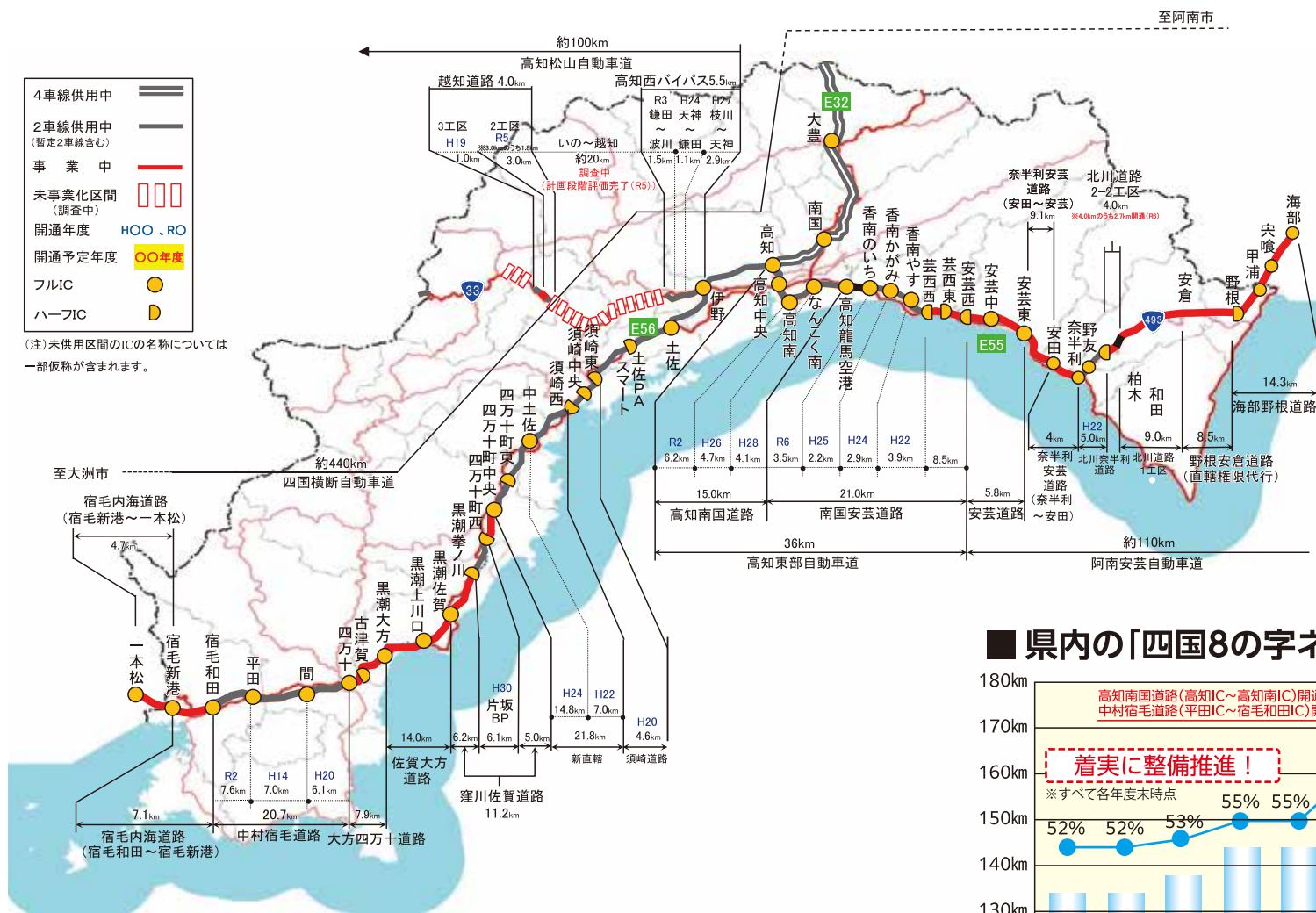
四国横断自動車道 窪川佐賀道路 (四万十町中央IC～四万十町西IC)
