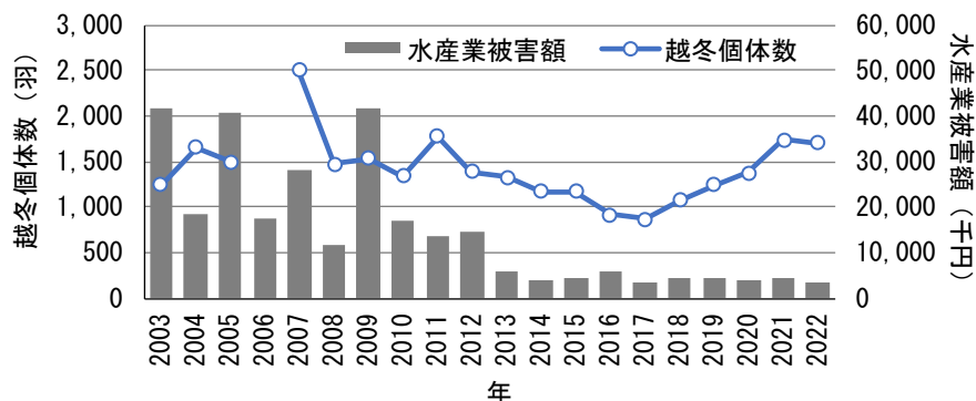
図 2-2-6 高知県におけるカワウの越冬個体数とカワウによる水産業被害額の推移
