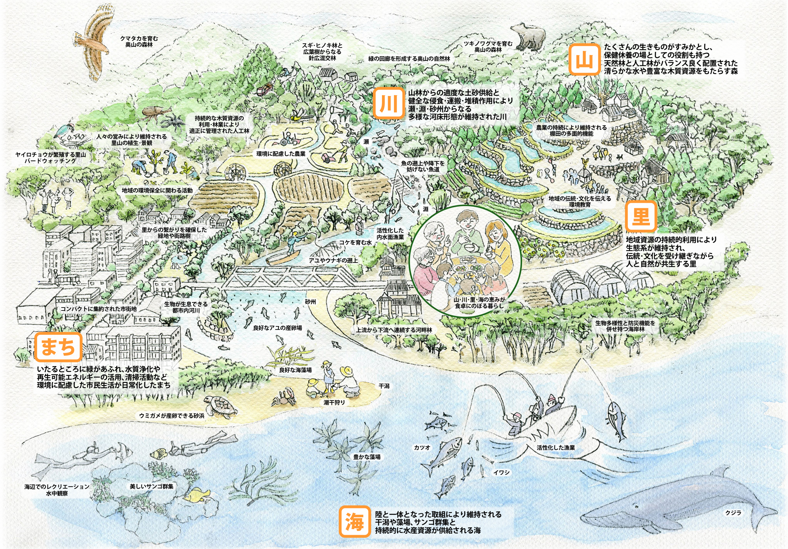
図 1-3-2 生物多様性こうち戦略によって目指すべき姿（イメージ図）
