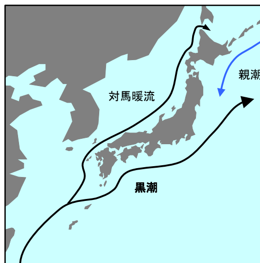
図 2-1-4 黒潮の流路
