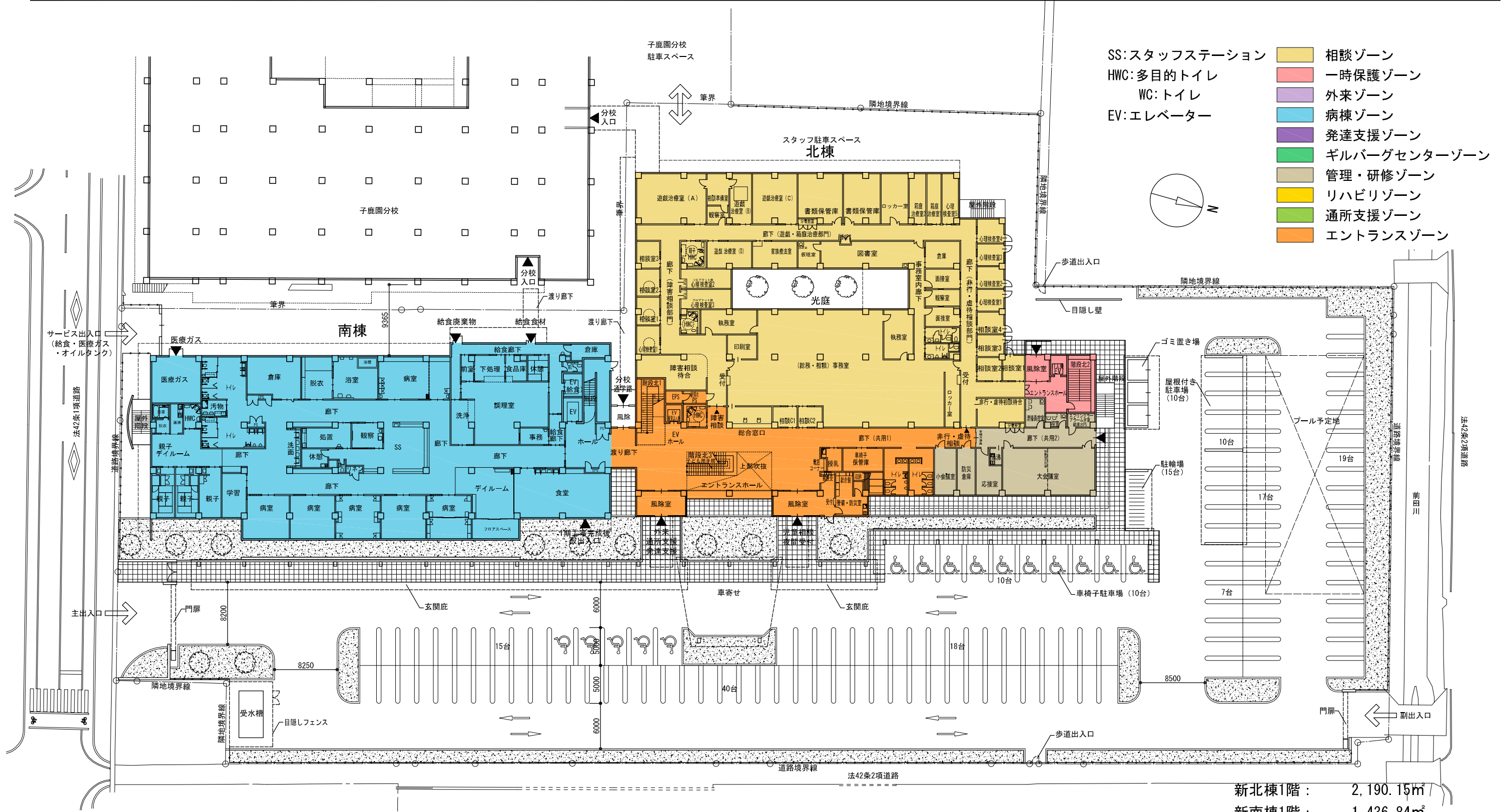
配置図兼 1階平面計画
