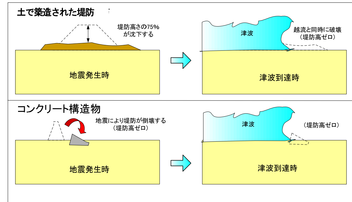
図 1-3-6 堤防の条件設定
